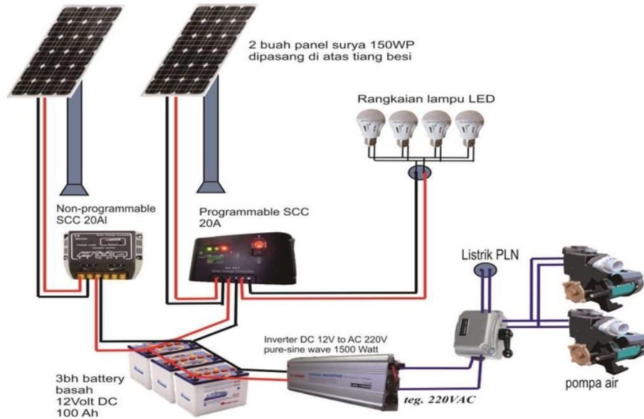
Gambar 1. Diagram Rangkaian Unit Pensuplai Daya Listrik Bertenaga Matahari
